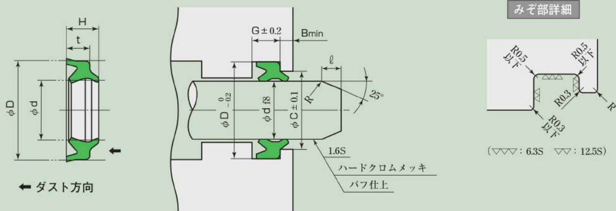
SDRスクレーパ寸法表
